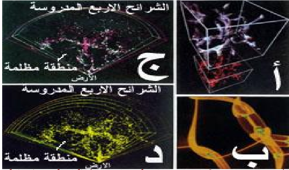
أ & ب : محاكاة بالحاسب الآلي لبناء التجمعات المجرية تشير إلى وجود الأربطة الكونية بين مناطق مظلمة ج & د : رسومات تخطيطية لأربع شرائح من سور المجرات العظيم وتبدو فيها المجرات والمناطق المظلمة العملاقة الفاصلة بينها
